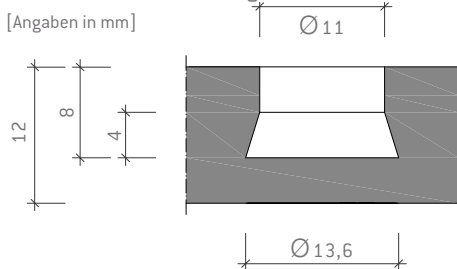
Bohrlochgeometrie Tergo+ Anker für 12 mm dicke [textura], [pictura], [natura] und [natura] PRO Tafeln Planung & Anwendung 2021
