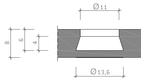
Bohrlochgeometrie Tergo+ Anker für 8 mm und 10 mm dicke [tectiva], [linea] und [lunara] Tafeln 67
