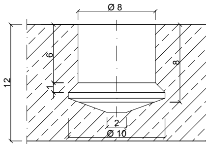
Bohrlochgeometrie Tergo Hinterschnittdübel [Angaben in mm]
