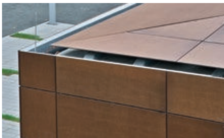
Gemeindeforum Ginsheim-Gustavsburg, Deutschland Gewinner des Deutschen Fassadenpreises 2011. Erdacht von Hille Architekten, fotografiert von Horst Goebel.
